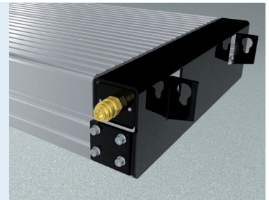
Druckluftversorgung 0016769
