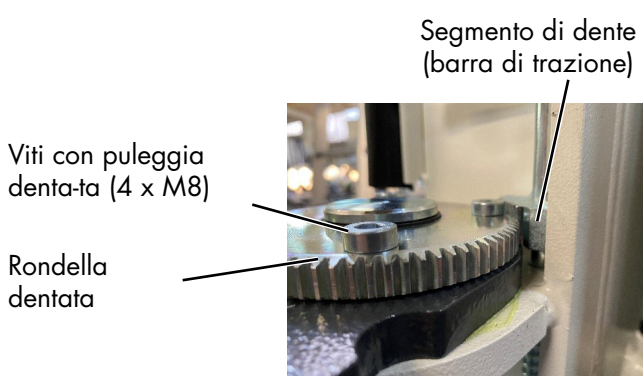
Agganciare i bulloni
